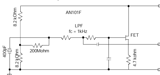
AN101F Inside Equivalent Circuit
