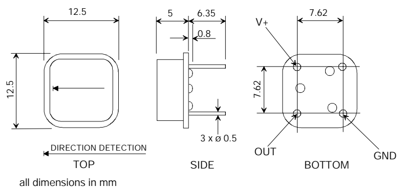
AN101 / AN101F Dimensions
